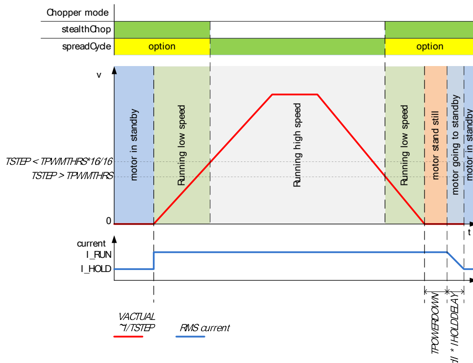
图 6.7 切换到 spreadCycle 的速度阈值 TPWMTHRS
