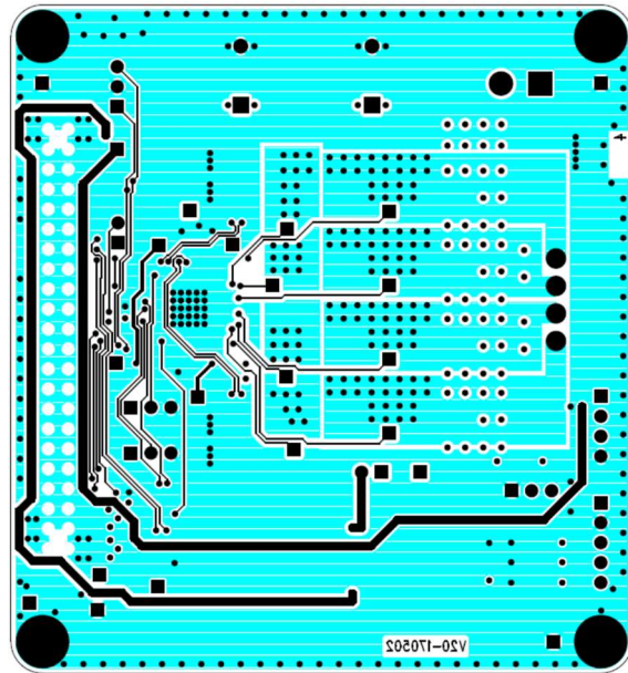
4- 底层
