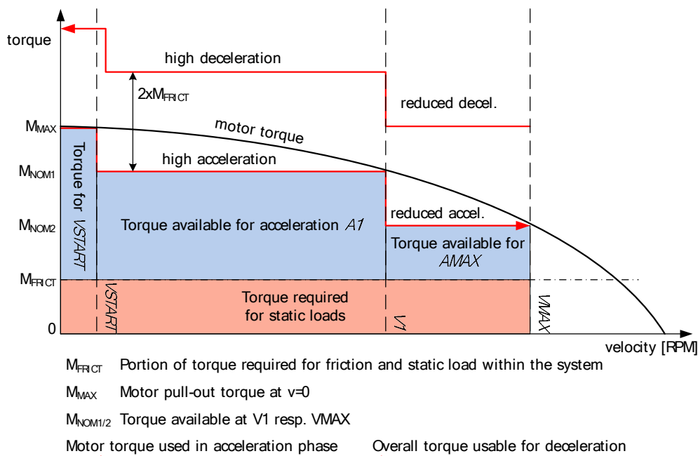
图 11.2 TMC5160 斜坡发生器优化电机转矩说明
