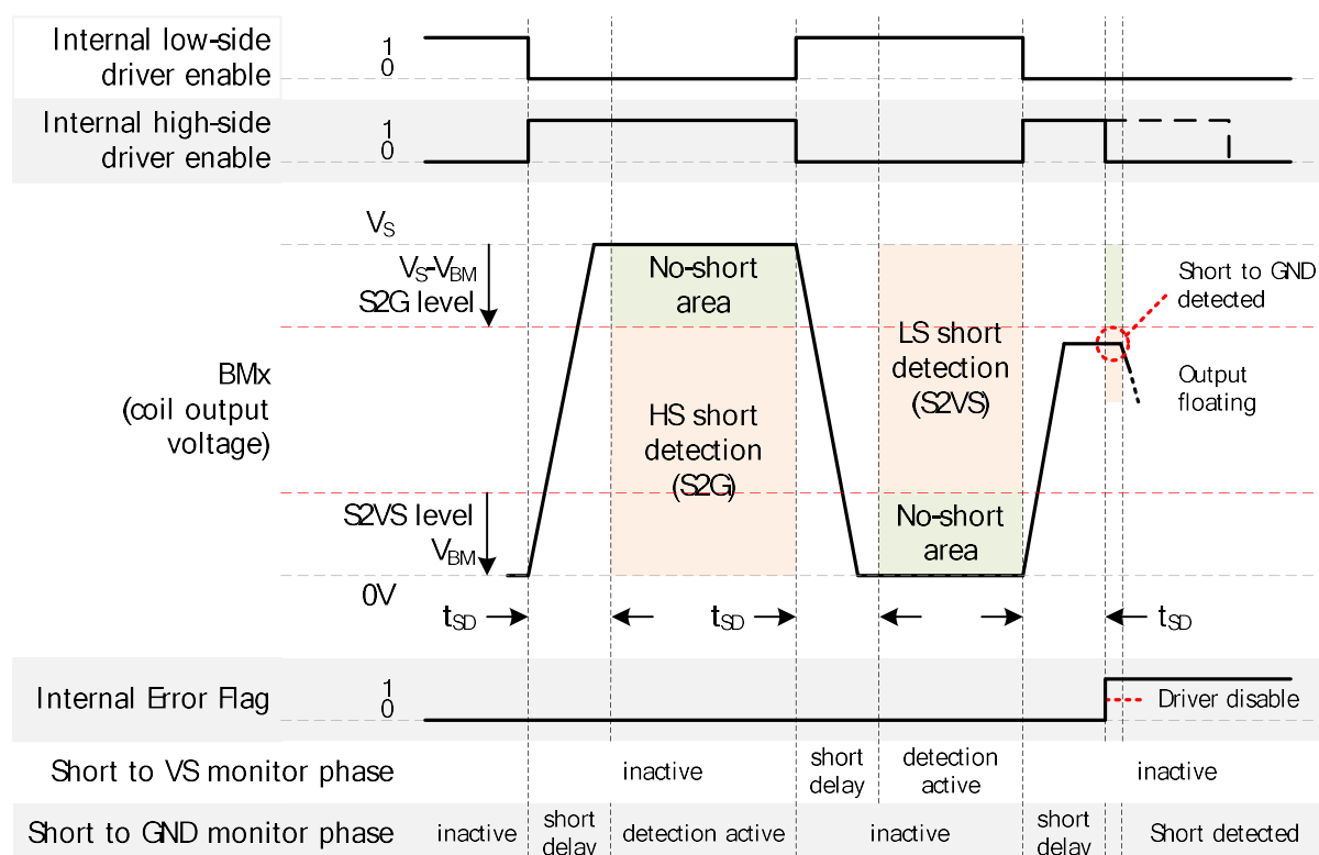
图 10.1 短路检测
