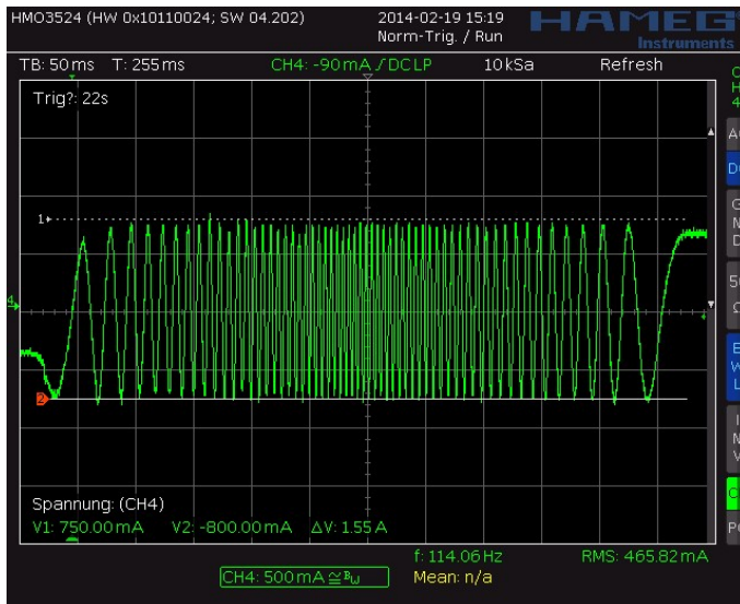
图 6.3 示波器: PWM_REG 优化设置
