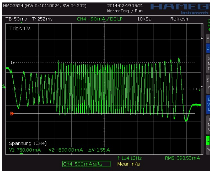
图 6.4 示波器:在 AT #2 期间, PWM_REG 的设置太小
